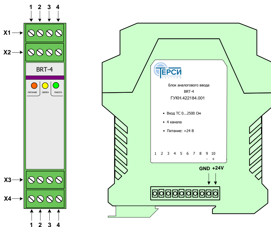
Рисунок 1 Внешний вид блока BRT-4 и расположение разъёмов
