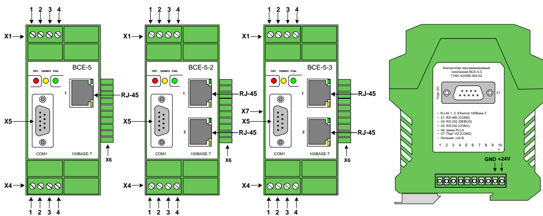
Рисунок 1 Внешний вид контроллера в различных исполнениях
