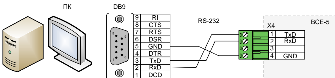
Рисунок 10 Схема подключения к отладочному порту контроллера
