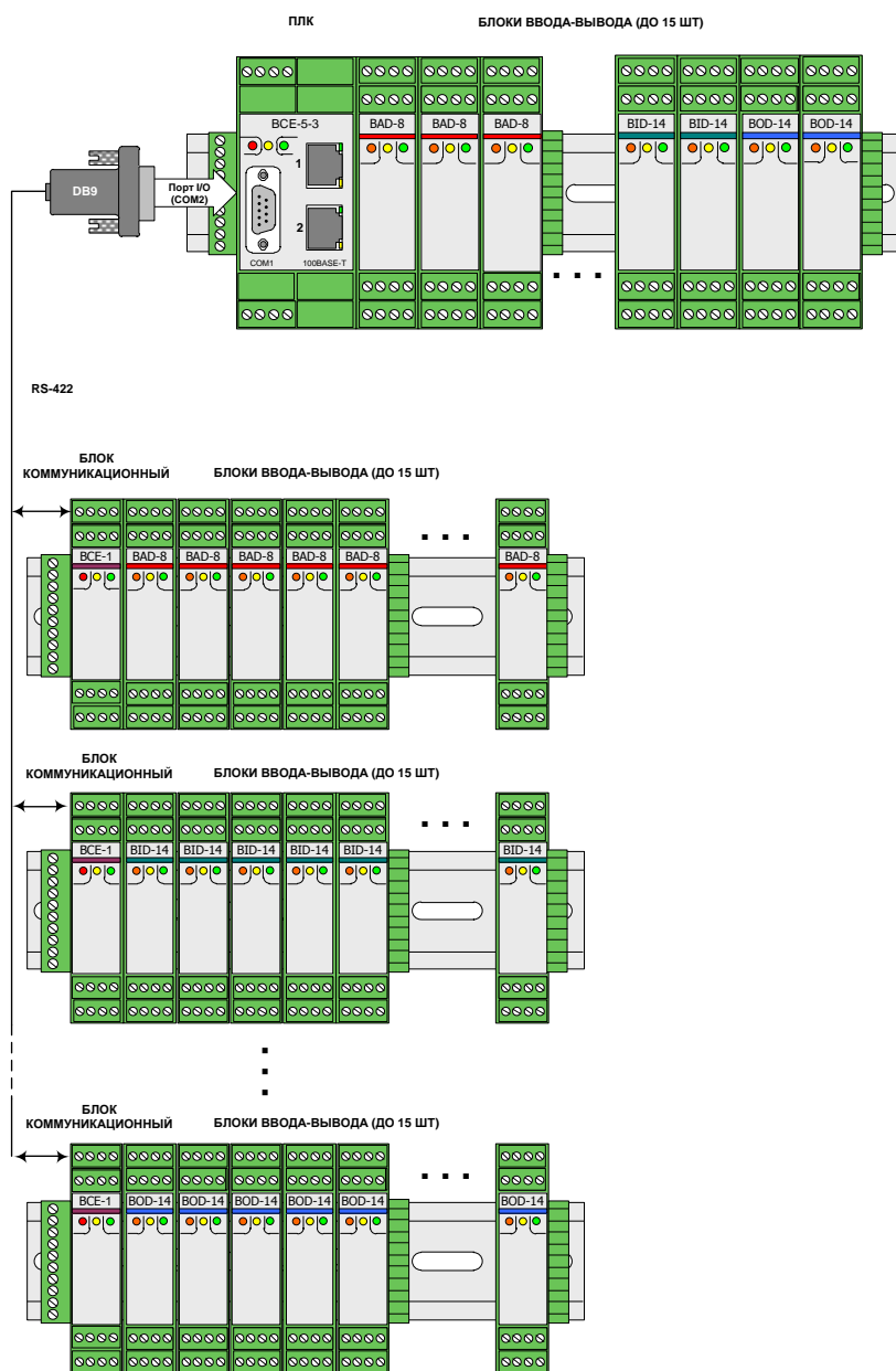
Рисунок 7 Пример подключения блоков ввода-вывода к контроллеру
