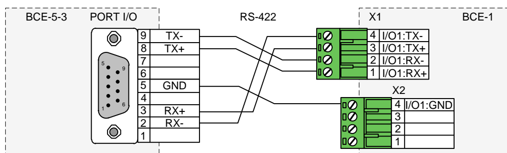
Рисунок 9 Схема подключения блоков ВСЕ-1 к порту I/O контроллера ВСЕ-5-3
