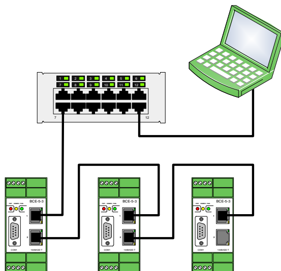
Рисунок 5 Подключение контроллеров при топологии «шлейф»
