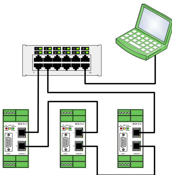
Рисунок 6 Подключение контроллеров при топологии «кольцо»
