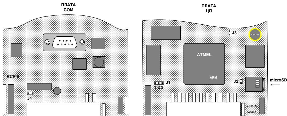
Рисунок 2 Расположение перемычек на плате контроллера
