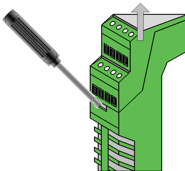
Рисунок 8 Извлечение платы контроллера из корпуса
